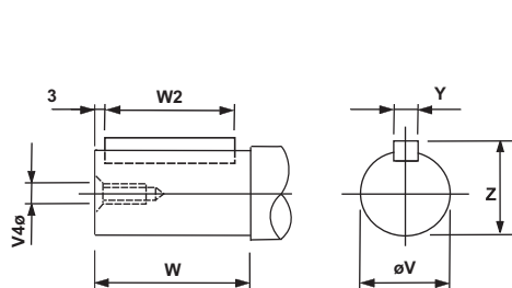
Input Shaft
