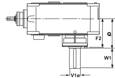
VB3 SA Heavy Duty Stirrer Drives
