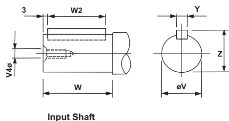
Input Shaft
