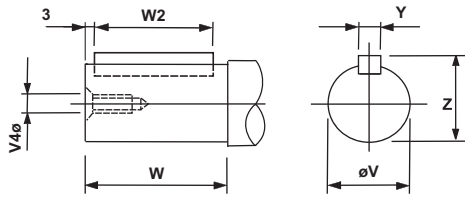
Input Shaft
