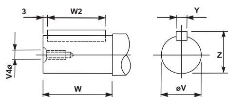
Input Shaft
