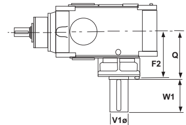
VB2 SA Heavy Duty Stirrer Drives
