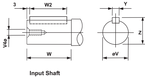
Input Shaft
